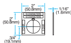
LP-40-SP POT
