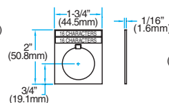
LP-43-SP POT
