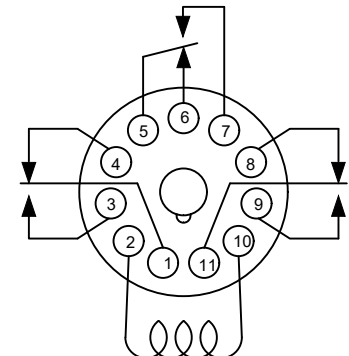
11 PIN 3PDT
